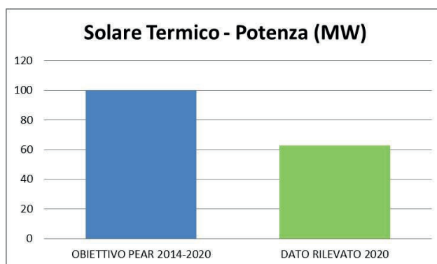
Figura 3-40 –Solare Termico, obiettivo e rilevato a confronto. Fonte: PEAR 2014-2020, GSE 2020
