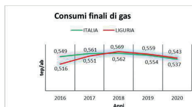
Figura 3-32 –Andamento elemento H “Consumi finali di gas” per Italia e Liguria anni 2016-2020 e grafico confronto procapite tep/ab. Elaborazioni a partire da dati GSE
