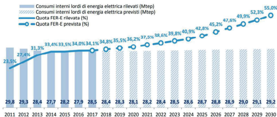
Figura 5-5 – Traiettoria della quota FER nel settore elettrico. Fonte: PNIEC
