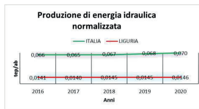
Figura 3-24 –Andamento elemento “Produzione di energia idraulica” per Italia e Liguria anni 2016-2020 e grafico confronto procapite tep/ab. Elaborazioni a partire da dati GSE
