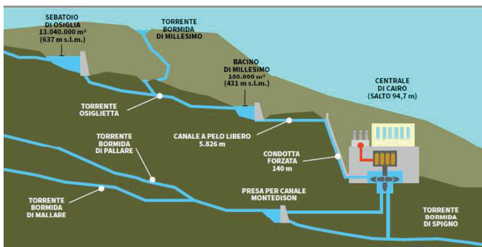
Figura 5-24 - Esempio di Centrale con invaso – Cairo Montenotte (SV). Fonte: Tirreno power
