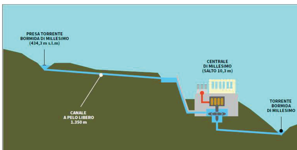
Figura 5-25 – Esempio di Centrale ad Acqua Fluente – Millesimo (SV). Fonte: Tirreno power
