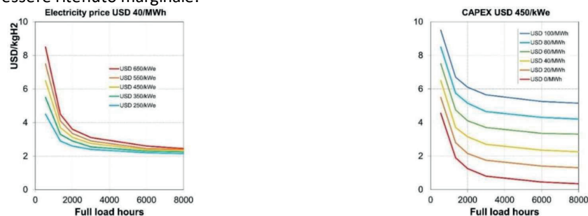
Figura 5-47 - Andamento del LCOE della produzione di idrogeno: A sinistra: LCOE al variare del CAPEX e del Load Factor; A destra: LCOE al variare del prezzo dell'elettricità e del load factor
