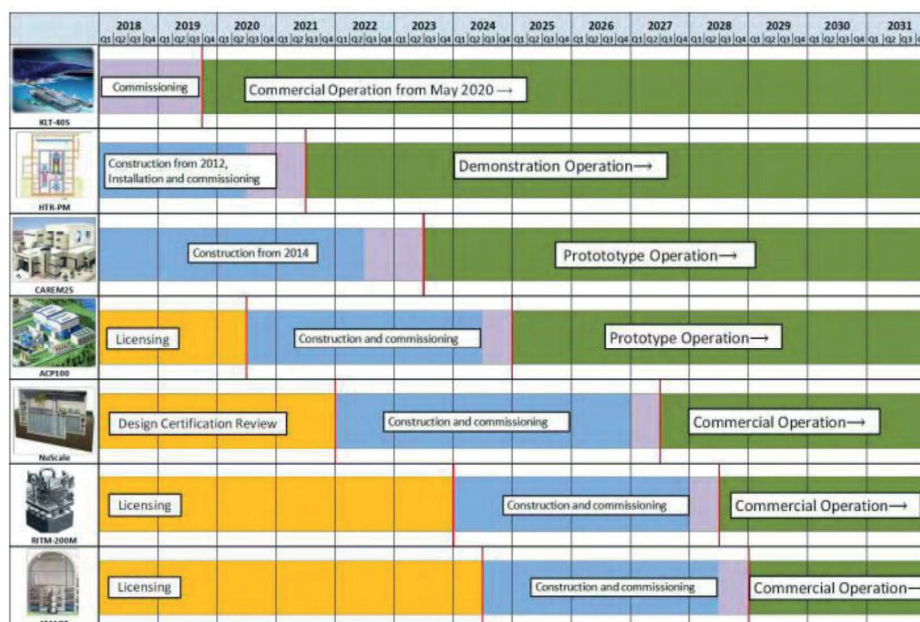
Figura 5-54 - Timeline dello sviluppo di alcuni SMR aggiornata al 2018
