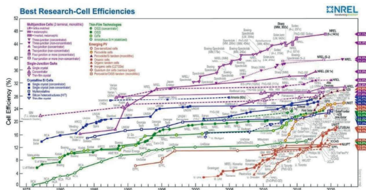
Figura 5-12 - Andamento storico dell'efficienza delle celle fotovoltaiche per tipologia di tecnologia 100
