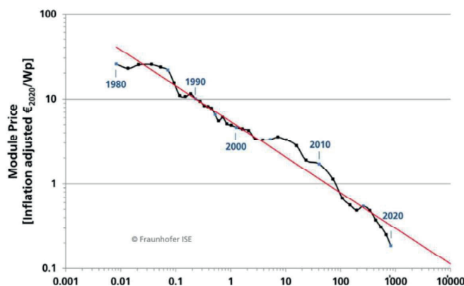
Figura 5-16 - Curva di apprendimento dei prezzi (price learning curve) rappresentativa di tutte le tecnologie PV disponibili sul mercato 109
