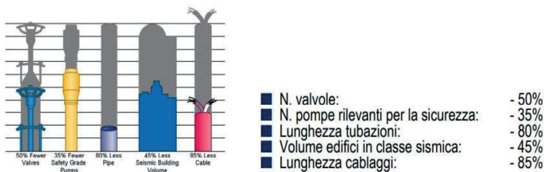
Figura 5-53 - Riduzione del numero di componenti nei PWR di III+ generazione (AP-1000 vs. PWR "classico") 201
