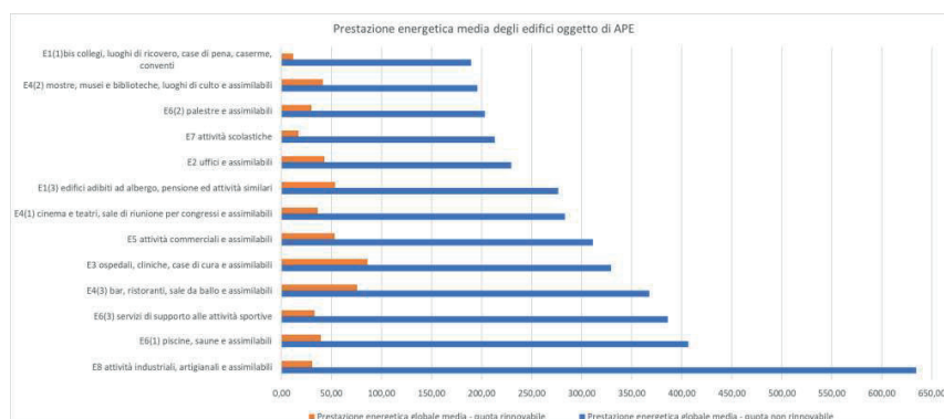
Figura 5-3 - Prestazione energetica globale media rinnovabile e non rinnovabile degli APE degli edifici non residenziali suddivisi per destinazione d'uso. Fonte: elaborazioni IRE SPA su Banca dati SIAPEL
