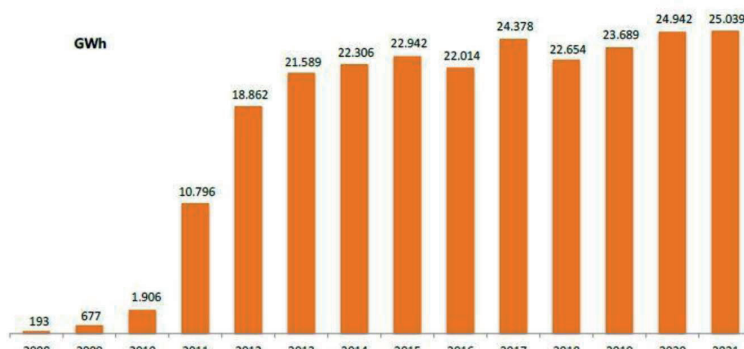
Figura 5-20 - Produzione annuale degli impianti fotovoltaici in Italia 114
