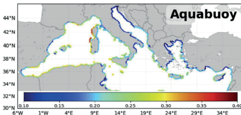
Figura 5-50 - Capacity factor per impianti di conversione dell'energia d'onda del tipo Single Aquabuoys 192
